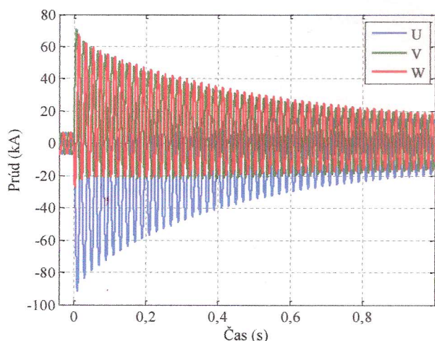
Obr. 5. Časový priebeh prúdov vo všetkých troch fázach pri vzniku ideálneho trojfázového skratu na svorkách synchronného generátora pri 100 % zaťaženi s účinníkom 0,485 indukčných.
