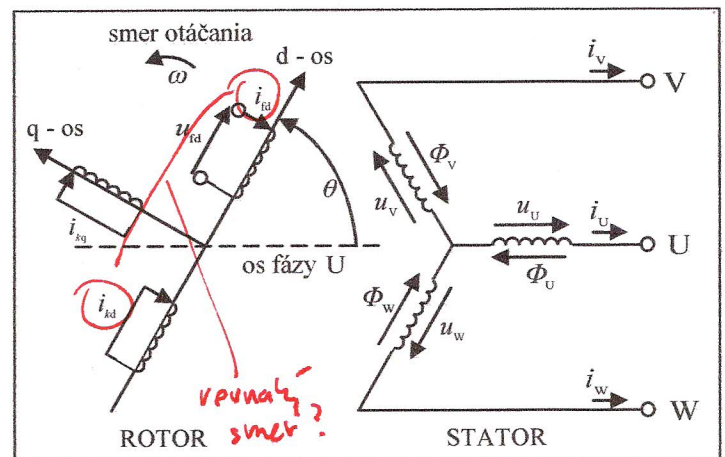
Obr. 1. Elektrické obvody rotora a statora synchronného generátora.
