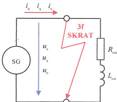
Obr. 2. Principiálna jedнопólová schéma zapojenia externej záťaže na svorky synchronného generátora (SG) s vyznačením vzniku ideálneho trojfázového (3f) skratu na svorkách SG.
